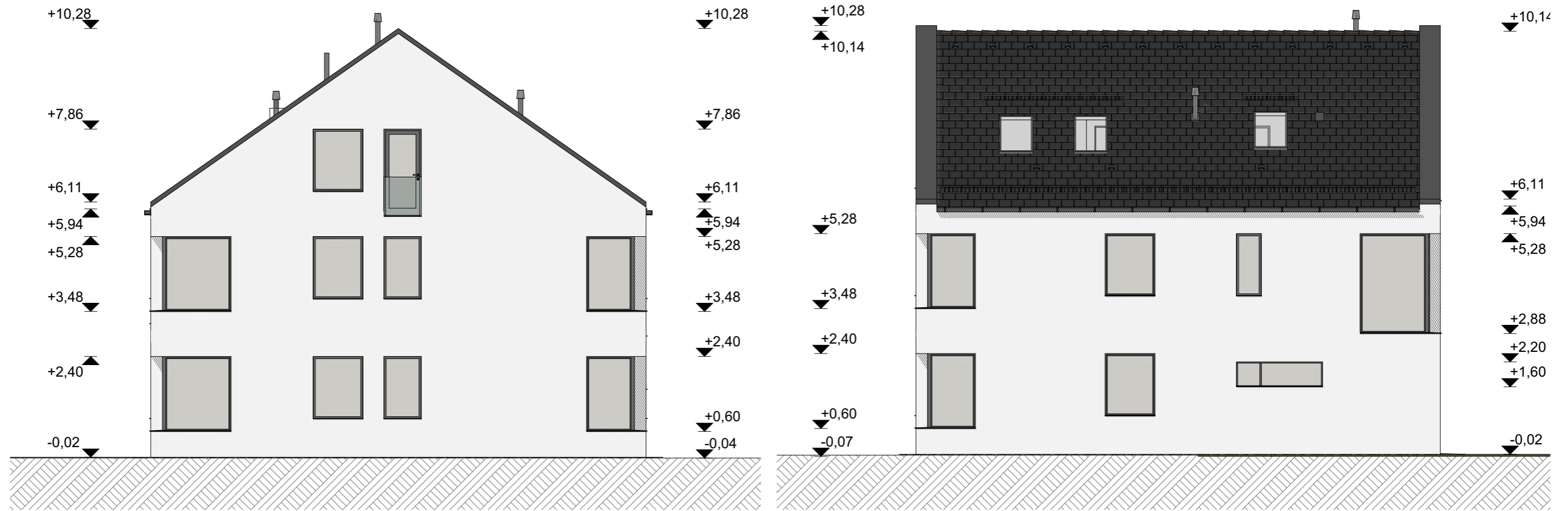
D homlokzat 1:100 K homlokzat 1:100
