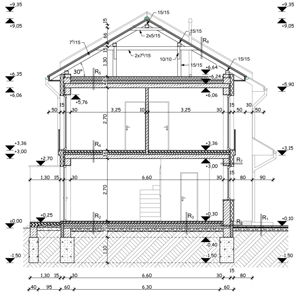
A-A metszet M=1:100
