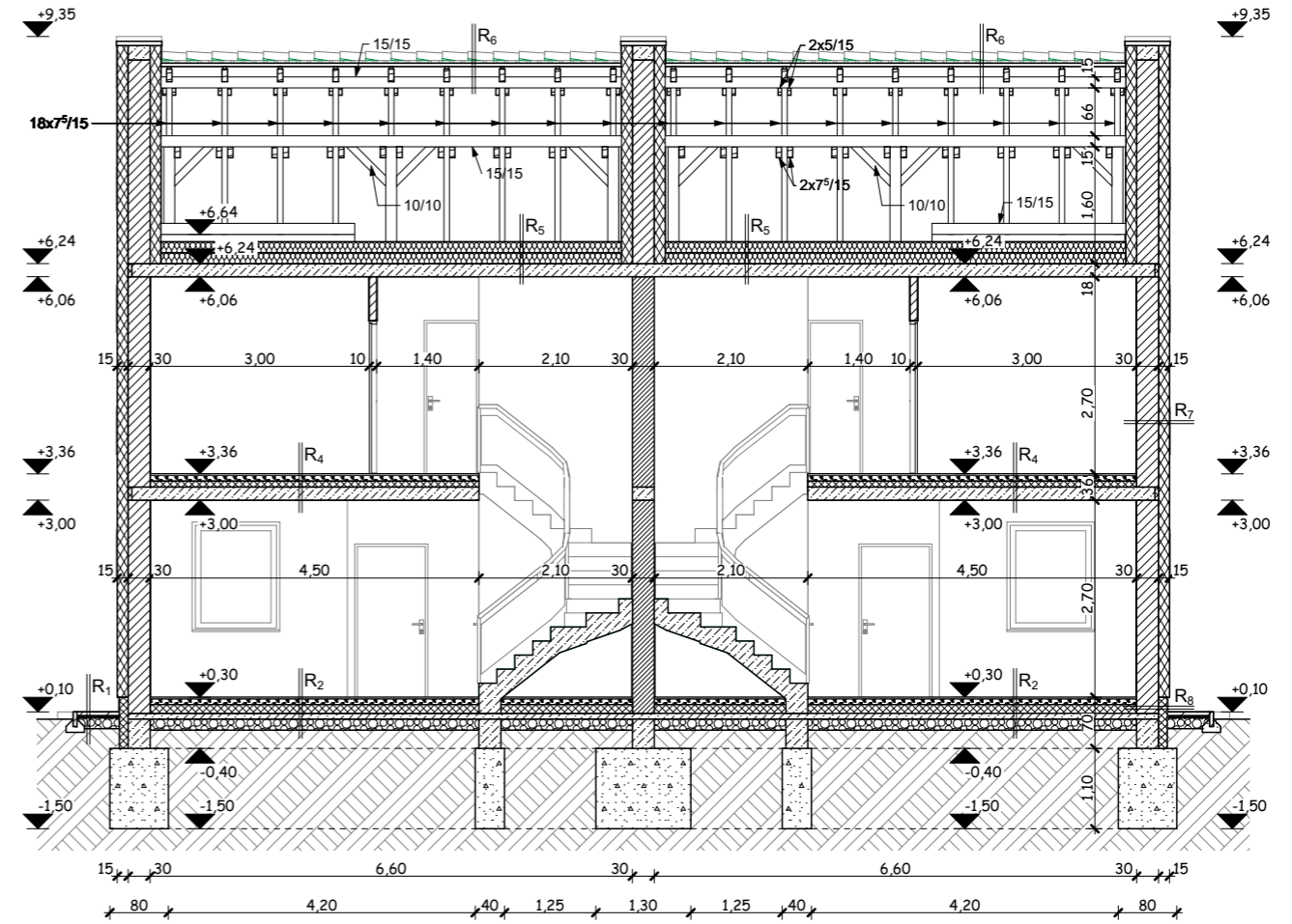
B-B metszet M=1:100
