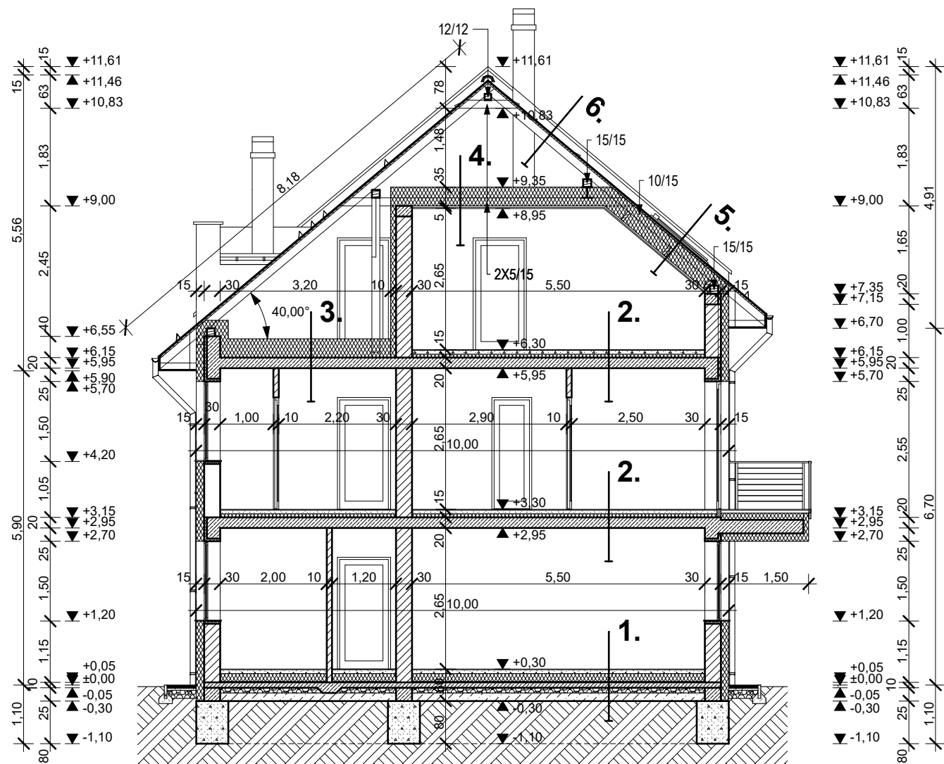
A-A METSZET M=1:100
